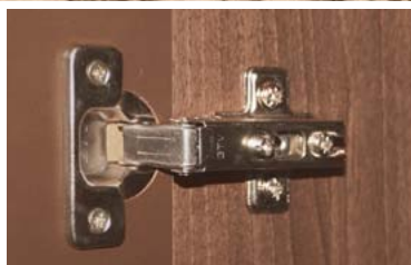
Zawiasy puszkowe \Phi 35mm regulowane w trzech płaszczyznach.
